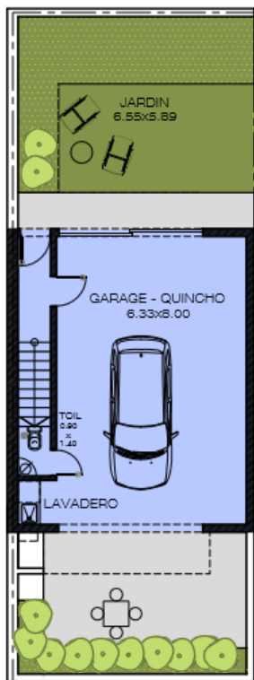
UF1 PLANTA BAJA
