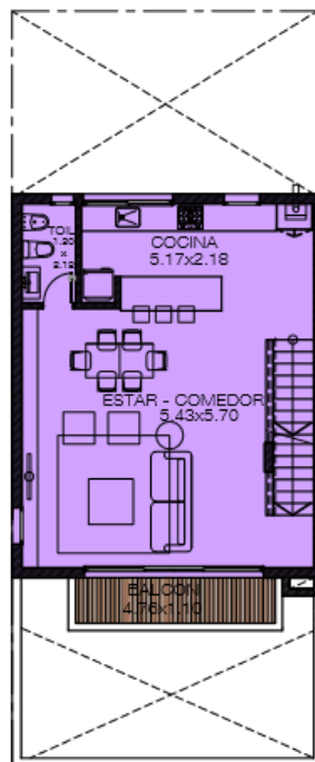
UF2 PRIMER PISO
