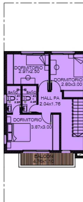
UF2 SEGUNDO PISO
