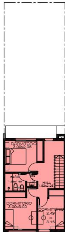
UF6 SEGUNDO PISO
