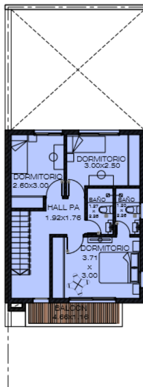
UF1 SEGUNDO PISO
